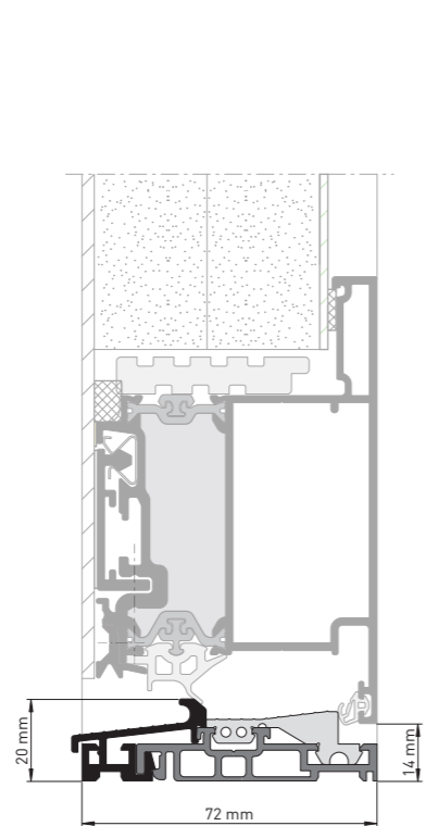
Durchlaufende Schwelle 2-teilig
